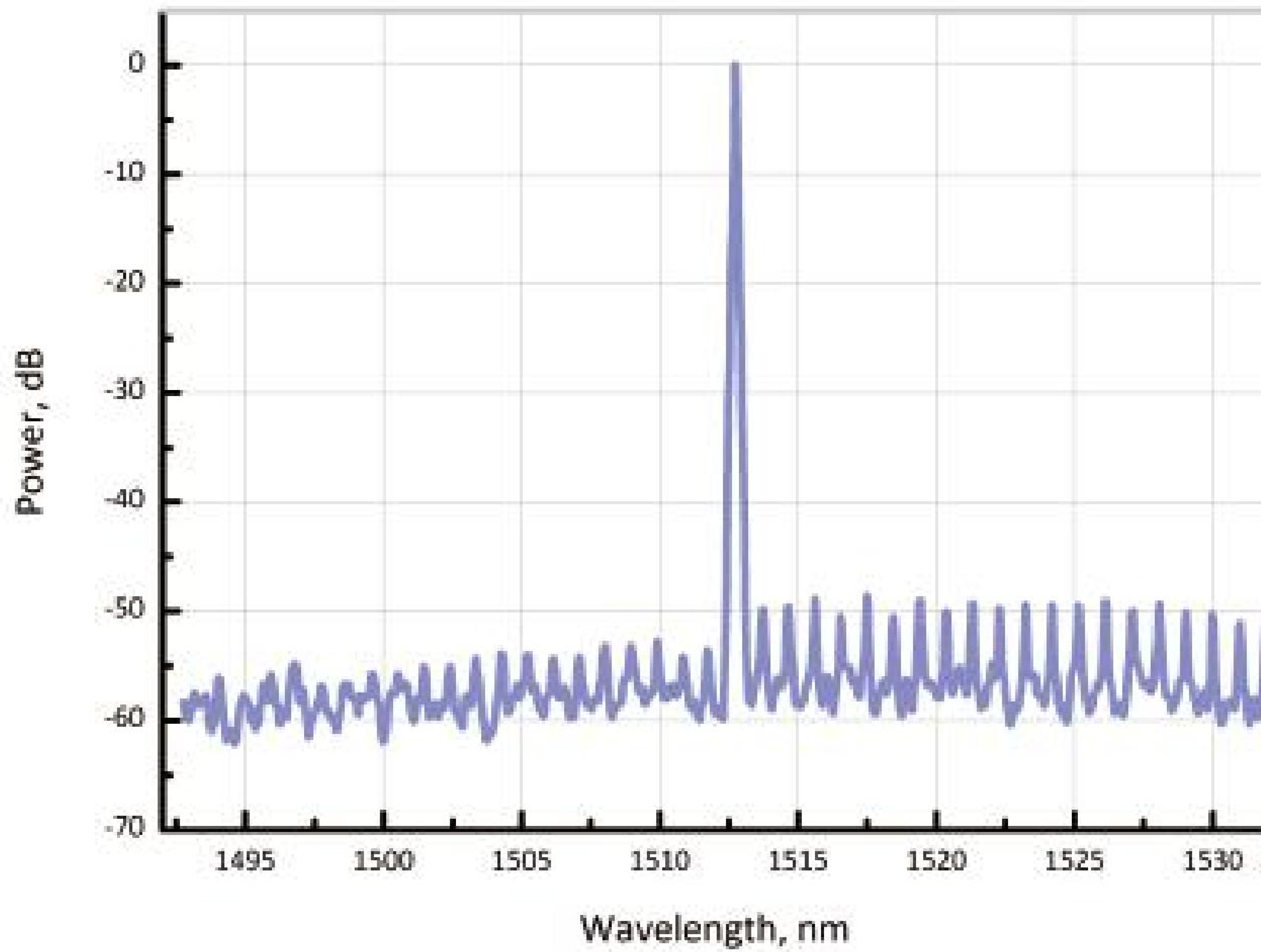
1512nm 可调谐模块测试图谱
